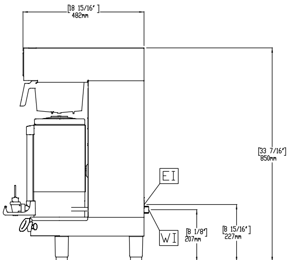
Zij aanzicht
